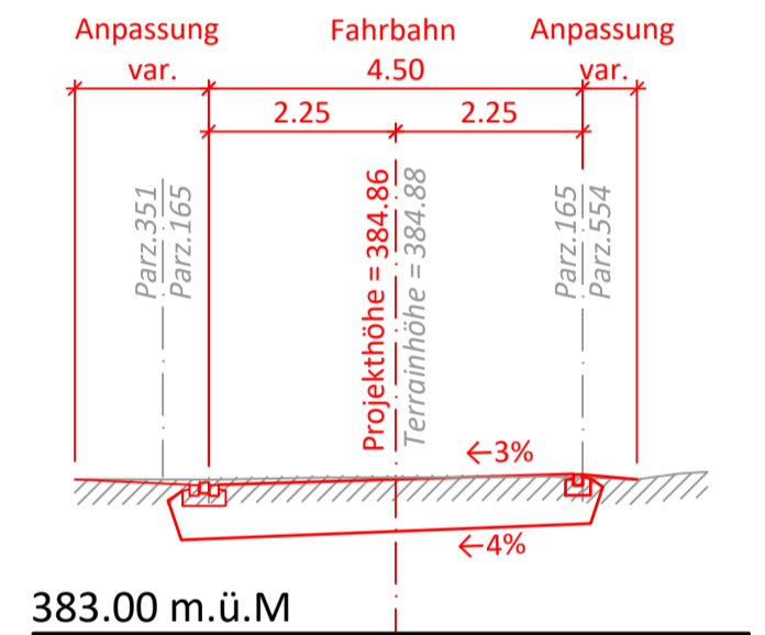
Querprofil 8, 30.00m
