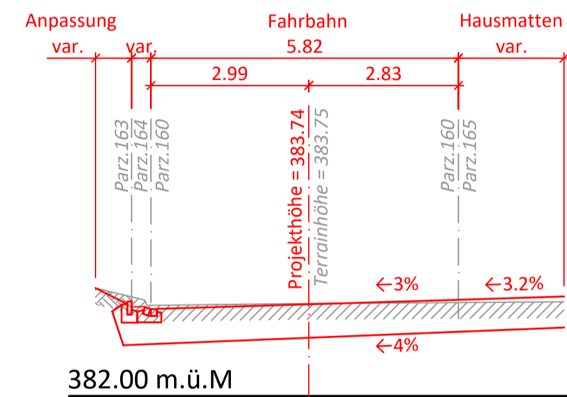
Querprofil 5, 125.00m
