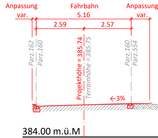
Querprofil 3, 75.00m
