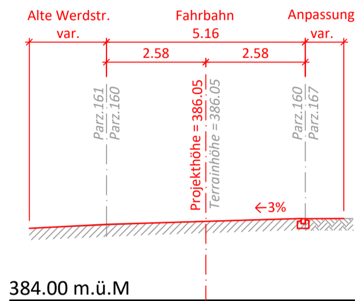
Querprofil 2, 50.00m
