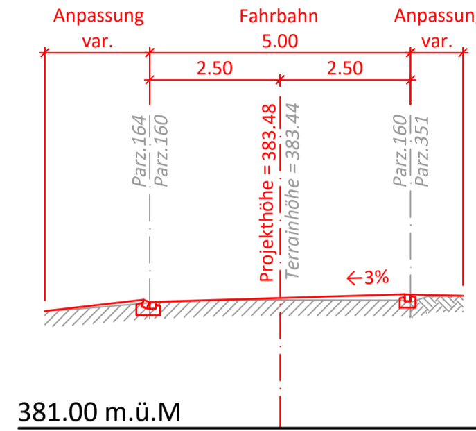
Querprofil 6, 134.00m
