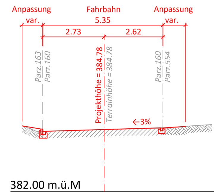
Querprofil 4, 100.00m
