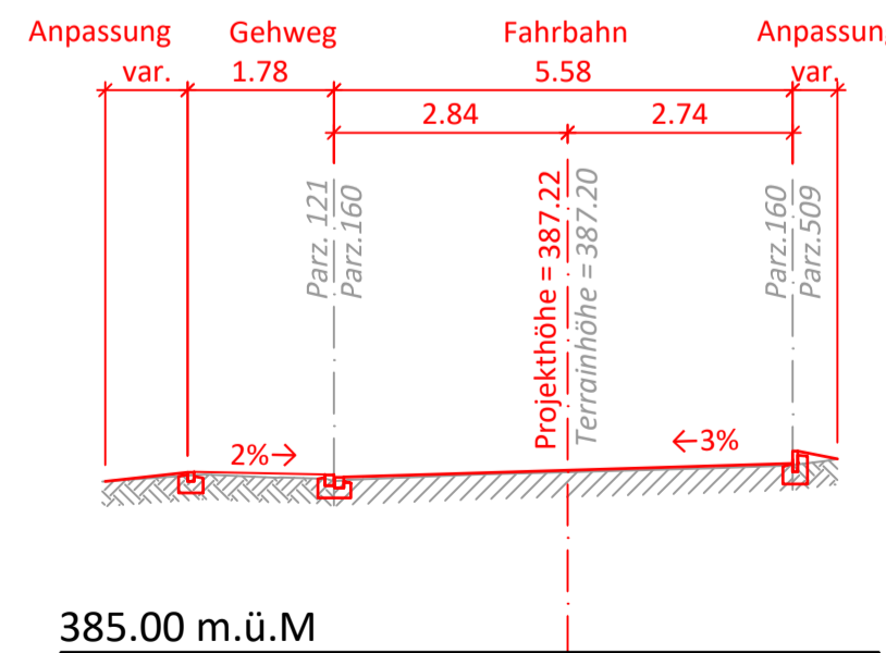
Querprofil 1, 20.00m
