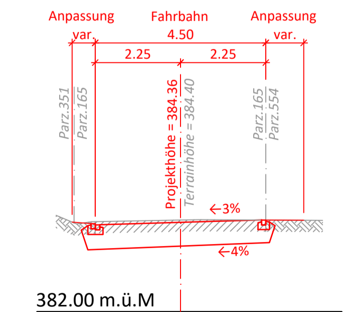
Querprofil 7, 15.00m
